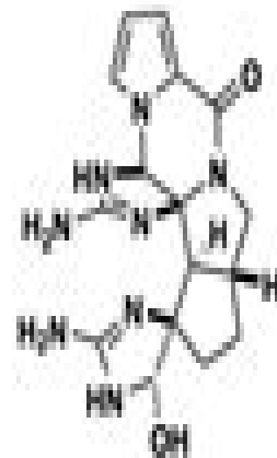
Palau'amine analog
