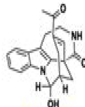
Tronocarpine
