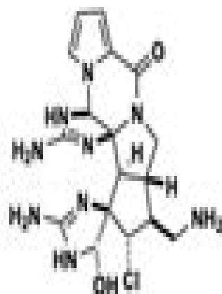
Palau'amine
