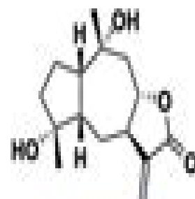
Guainolides
