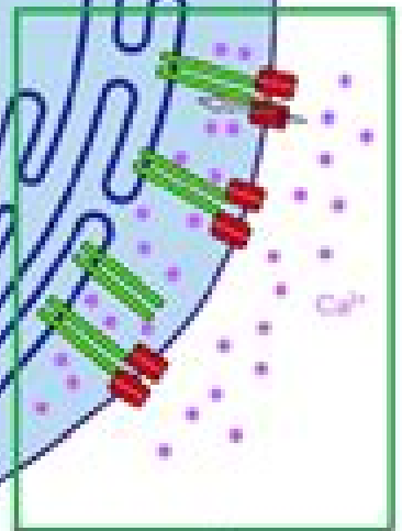
Empty \text{Ca}^{2+} -store in ER-lumen
