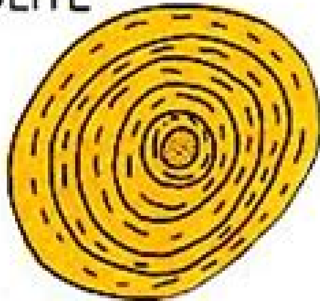
ARAGONITE OOLITE
