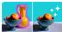
Erase & Replace
