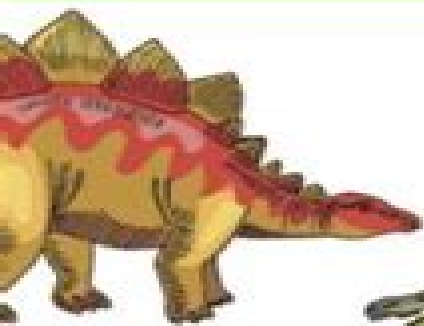
STEGOSAURUS
