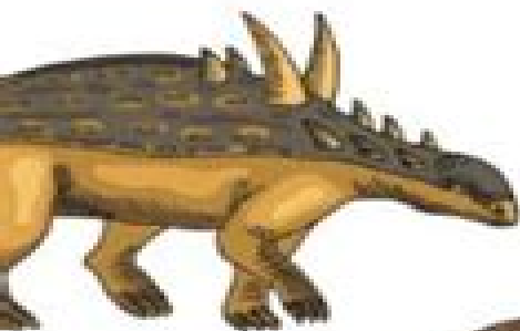
ACANTHOPHOLIS
