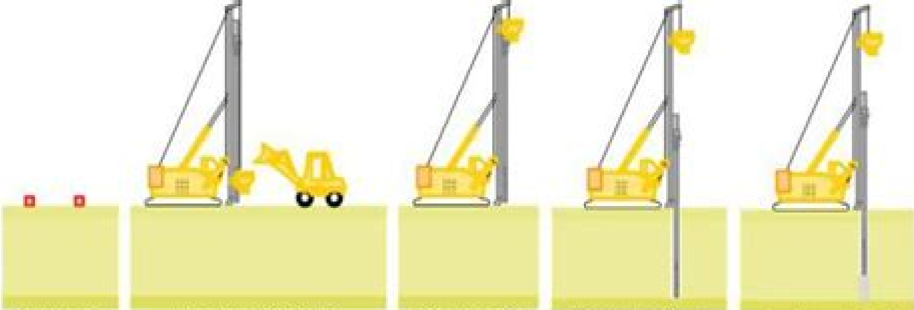
Plateforme et implantation
