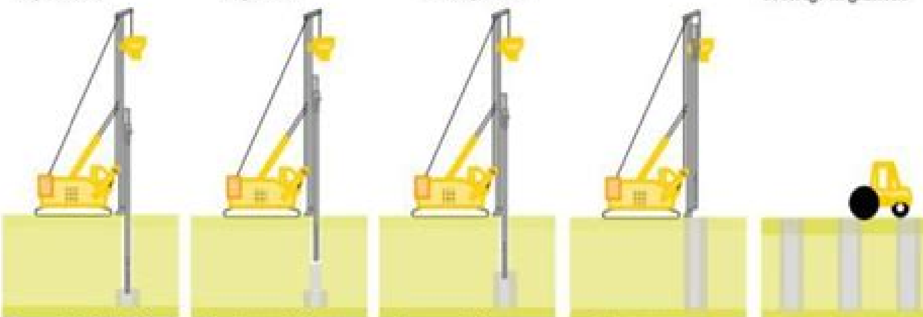
Bourrage du ballast dans le sol par vibration
