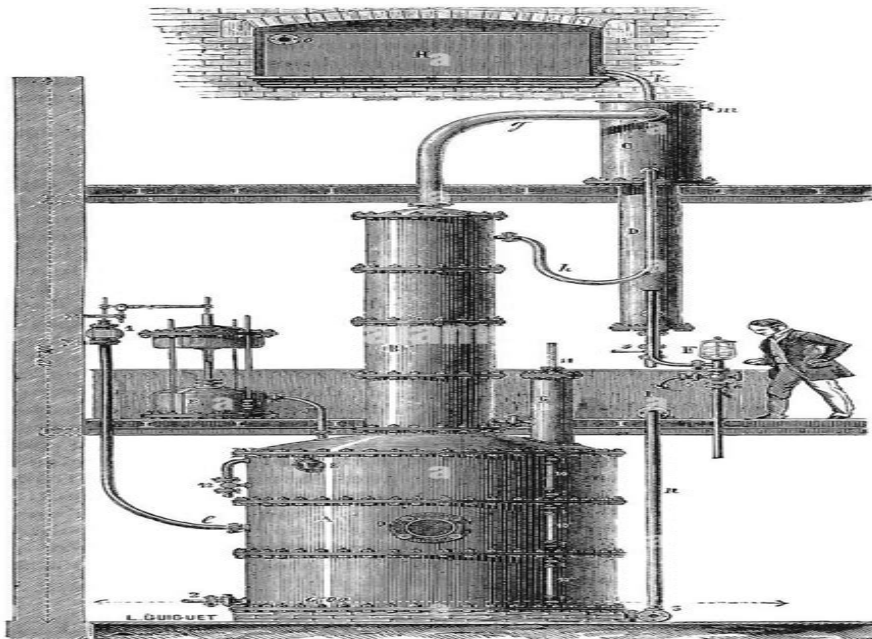
Fig. 288. — Appareil de rectification des alcools de M. Désiré Savalle.
