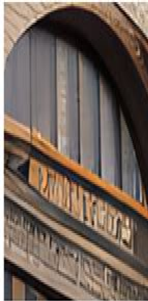
R-ESRGAN
