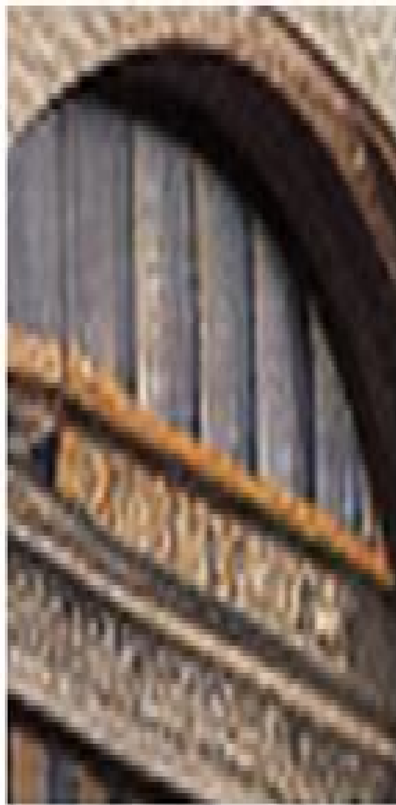
Lanczos
