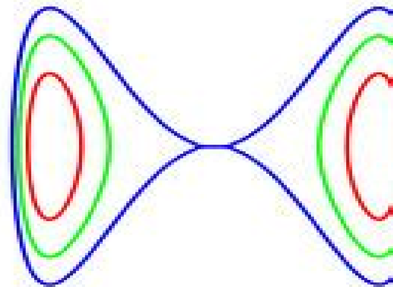
(d) "Figure eight cuspidal-loop"
