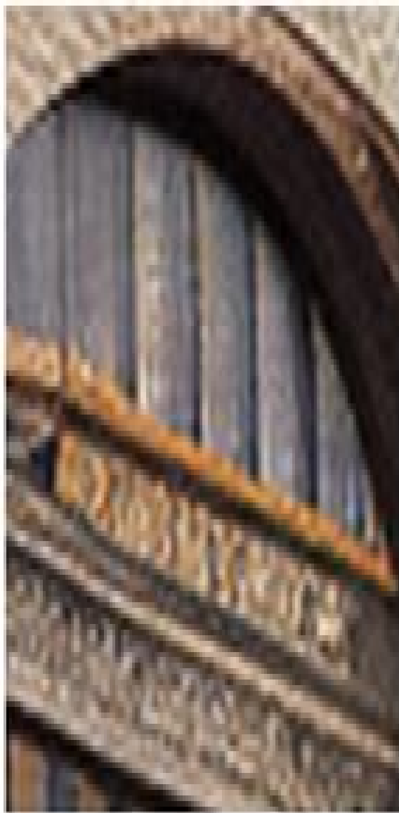
Lanczos
