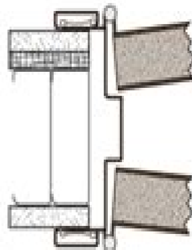
18 Jamb Hinge/Hinge
